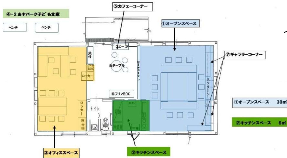
施設平面図
